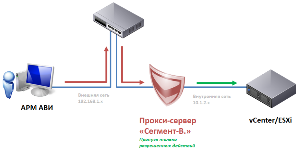
Рисунок 1 - Схема организации сети при использовании «Сегмент-В.»
