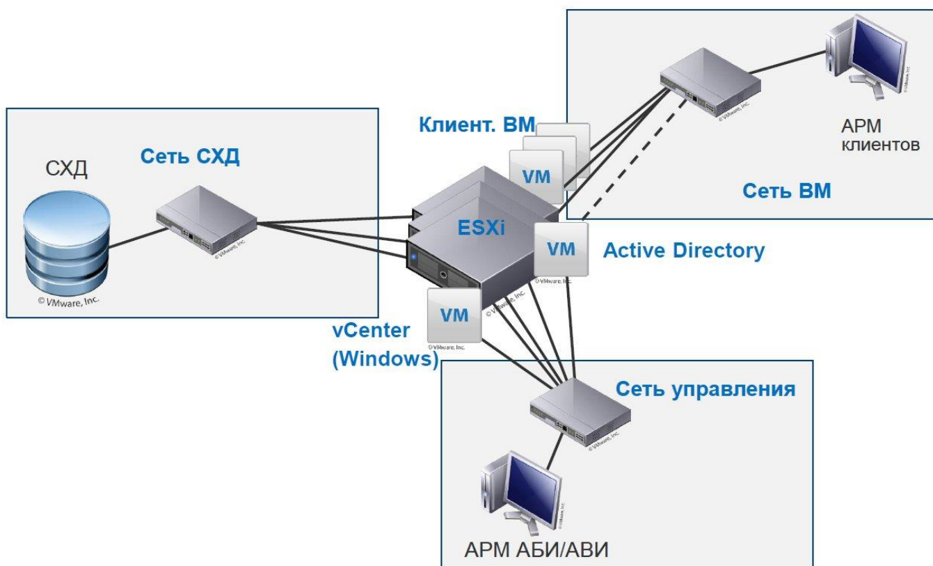
Рисунок 2 - Пример развертываемой инфраструктуры
