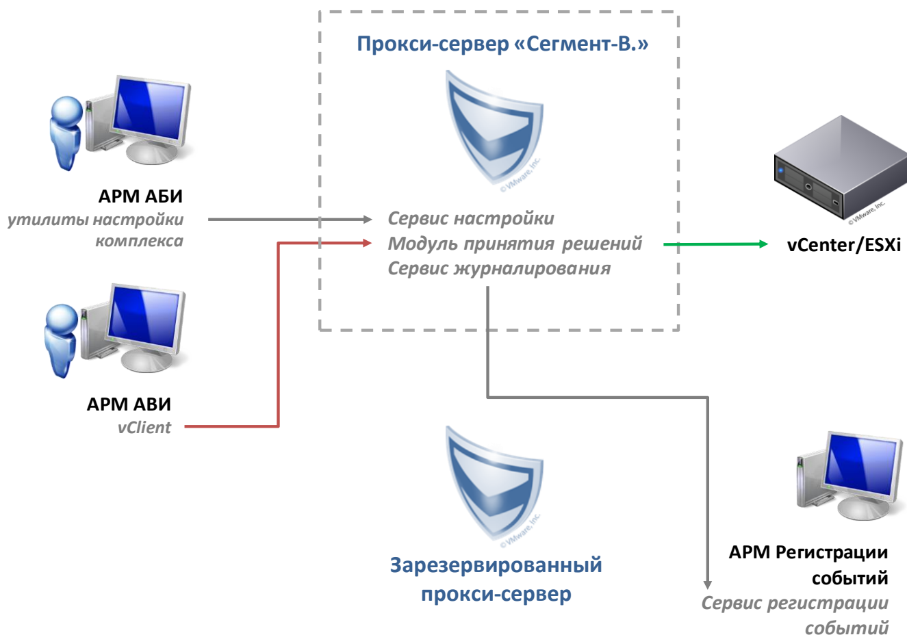
Рисунок 3 - Общая схема решения
